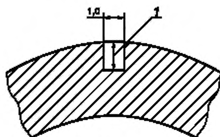
1 — глубина надреза
