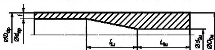
а — Внутренняя высадка, все группы прочности
