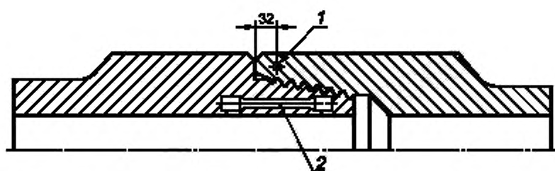
а — Участок контроля твердости муфты и расположение образца для испытания на растяжение для ниппеля
