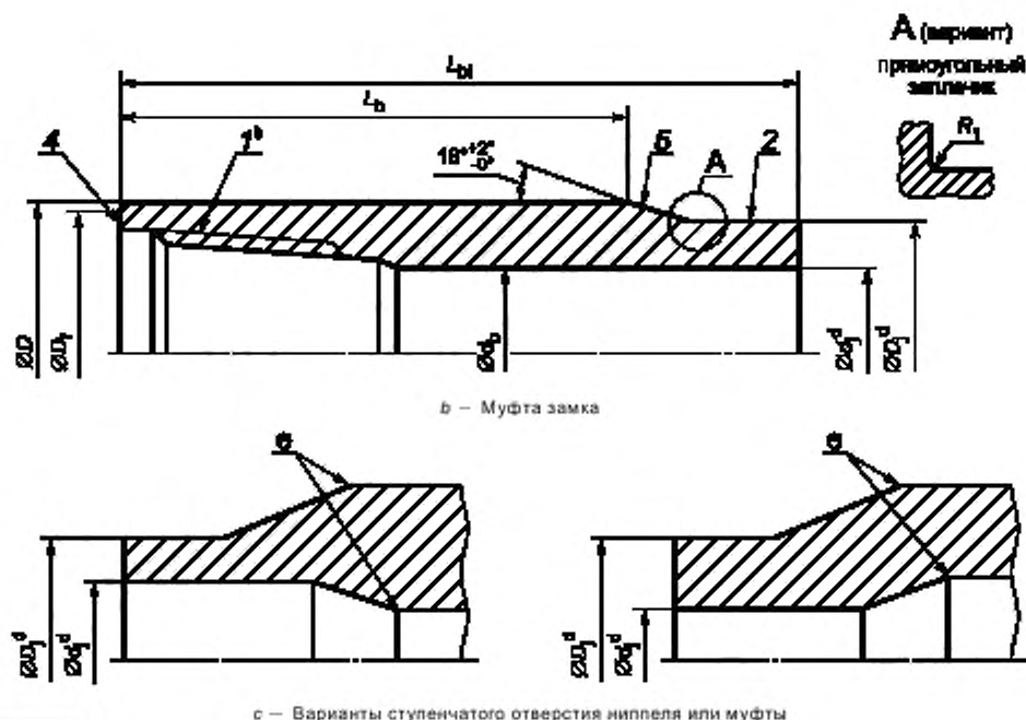
с — Варианты ступенчатого отверстия ниппеля или муфты
