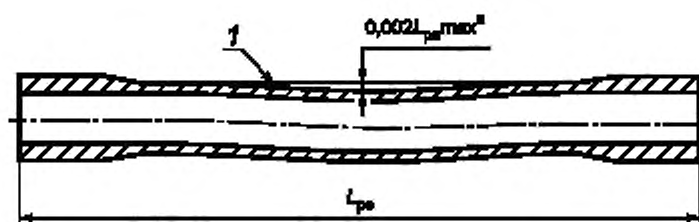
a — Измерение общей прямолинейности
